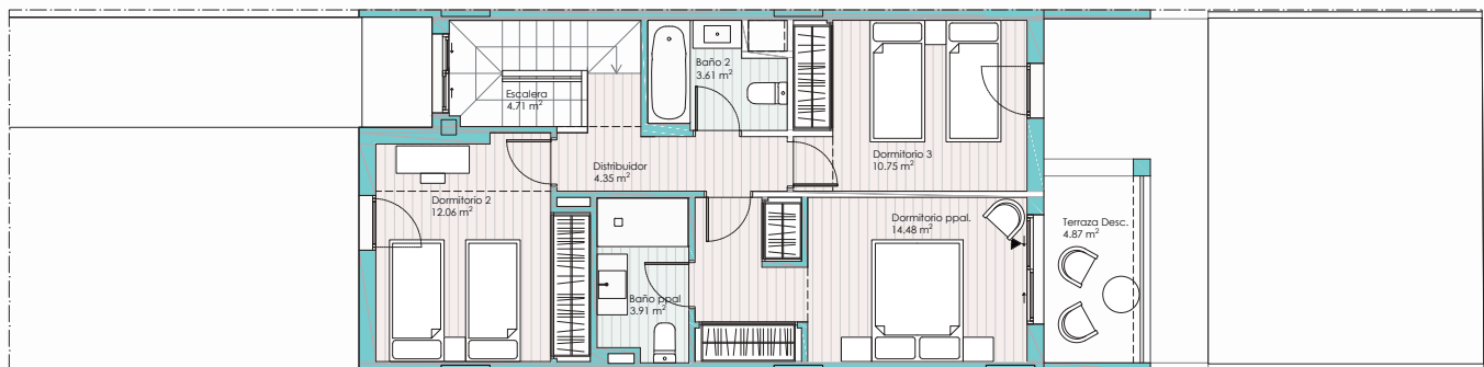
Planta Alta
