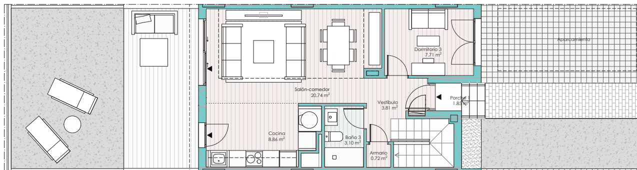
Planta Baja
