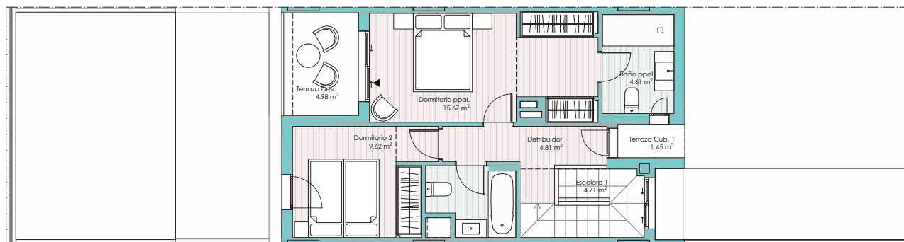
Planta Alta
