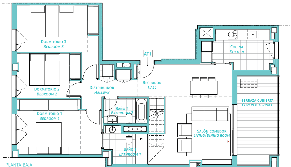
PLANTA BAJA
